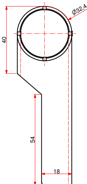
101A0340K - PIPA DESTRA 45X110 SCARICATA - PP - Nat.
