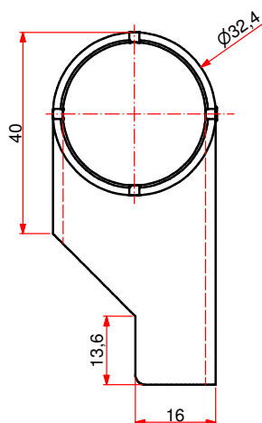
101A0343G - PIPA DESTRA 45X70 SCARICATA - PP - Nat.
