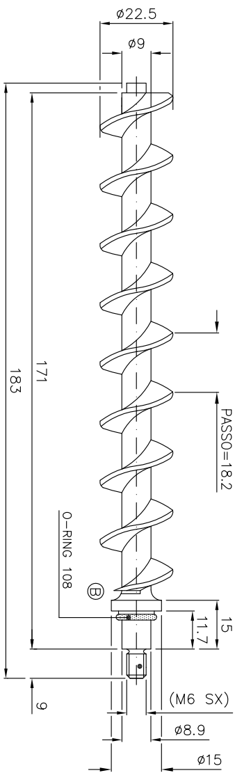
COCLEA TIPO NUOVO Cod. 201A0510H
