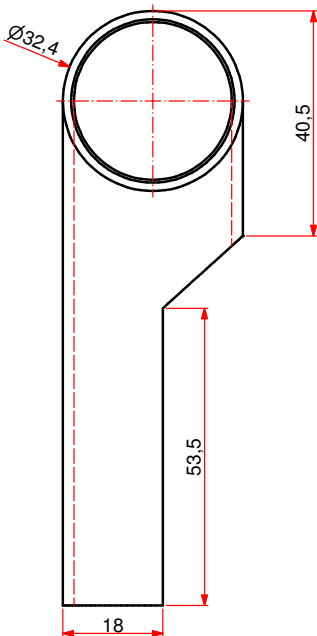
101A0341A - PIPA SINISTRA 38x107 - PP - Nat.
