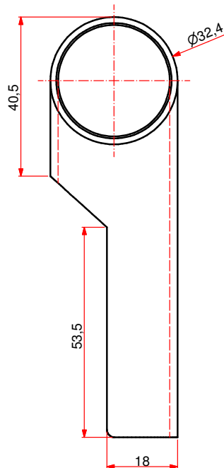
101A0340A - PIPA DESTRA 38x107 - PP - Nat.
