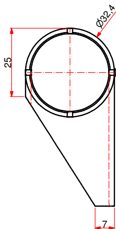
101A0343F - PIPA DESTRA 45X65 SCARICATA - PP - Nat.
