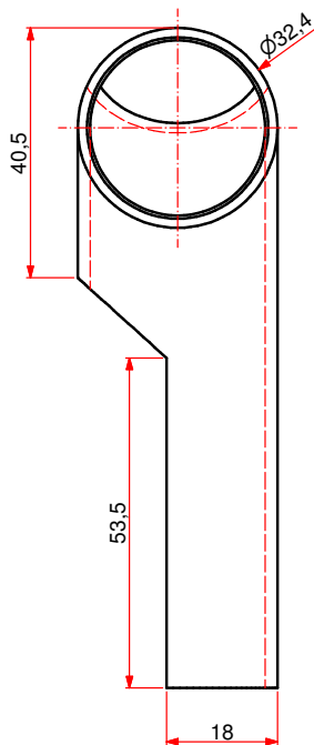
101A0340B - PIPA DESTRA 38x107 C/CAMINO - PP - Nat.
