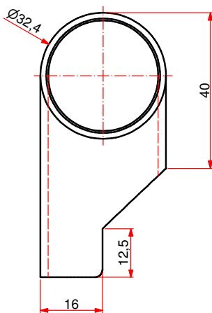
101A0345A - PIPA SINISTRA 38x68 - PP - Nat.
