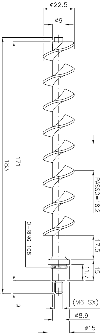
COCLEA TIPO VECCHIO Cod. 201A0510B
